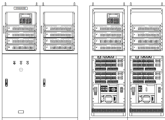
定刻起床装置集中型（128床タイプ） SMC-2, SMC-3
