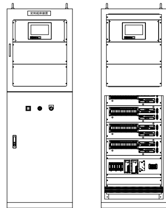
定刻起床装置集中型（64床タイプ） SMC-3-1
