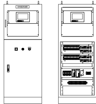
定刻起床装置集中型（32床タイプ） SMC-3-1
