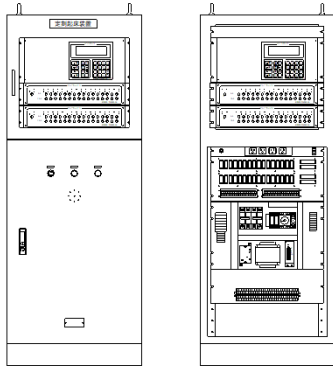
定刻起床装置集中型（32床タイプ） SMC-2, SMC-3
