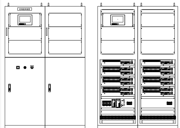
定刻起床装置集中型（128床タイプ） SMC-3-1
