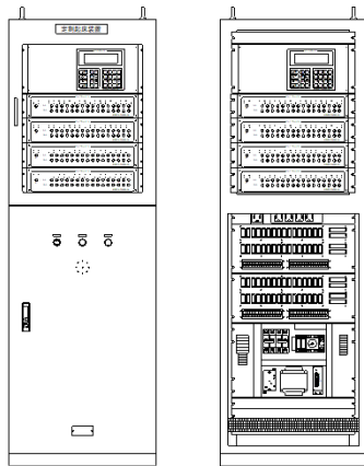
定刻起床装置集中型（64床タイプ） SMC-2, SMC-3
